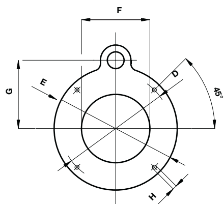
Foratura piastra bruciatore per Cosmo aluFer (200-950)
